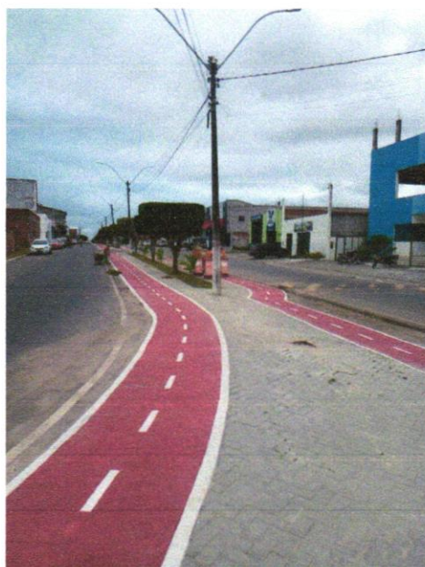
Foto 10 - PINTURA DE PISO COM TINTA ACRÍLICA, APLICAÇÃO MANUAL, 2 DEMÃOS, INCLUSO FUNDO PREPARADOR. AF05/2021
