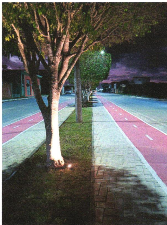
Foto 03- Pavimentação em bloco de concreto vibroprensado, intertravado, cor natural, 10x20cm, e=6cm, 46un/m 2 , NBR9781, Fck(min)=35MPa, sob coxim areia grossa compactada c/ placa vibratória, e(comp.)=6cm, rejuntado c/ areia fina.
